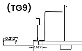
9/16" T-BAR
