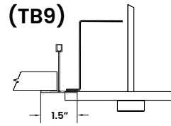
9/16" T-BAR
