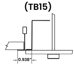
15/16" T-BAR
